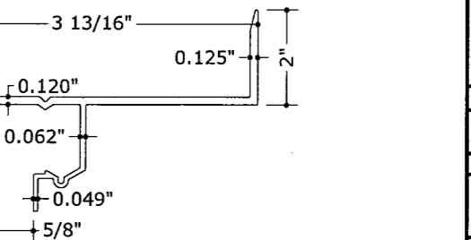
39 ALT. BUILD-OUT WALL HEADER N.T.S. 6063-T6
