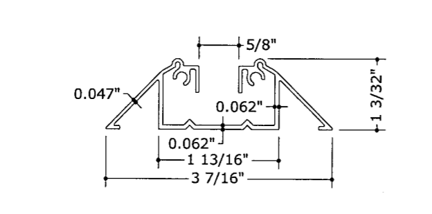
16 WALKOVER TRACK N.T.S. 6063-T6
