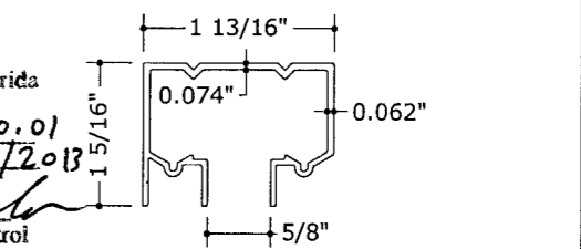
37 ALT. CEILING HEADER N.T.S. 6063-T6
