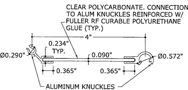
2 WINDOW BLADE N.T.S. 6063-T6/POLYCARBONATE
