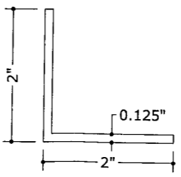
35 2"x2"x0.125" ANGLE N.T.S. 6063-T6
