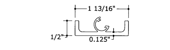
31 CEILING SIDE MOUNT N.T.S. 6063-T6
