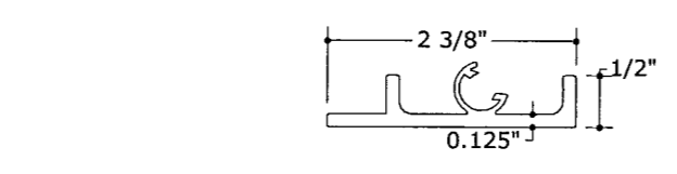
32 HEADER SIDE MOUNT N.T.S. 6063-T6
