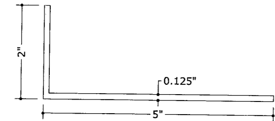
27 2"x5"x0.125" ANGLE N.T.S. 6063-T6
