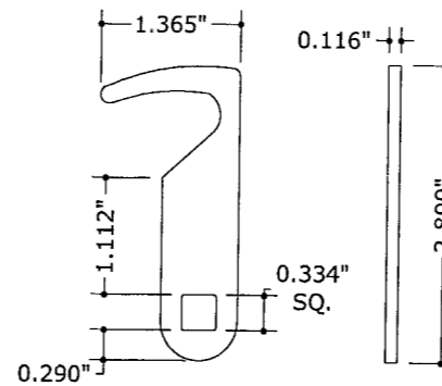
24 LOCKING ARM N.T.S. 410 STAINLESS STEEL
