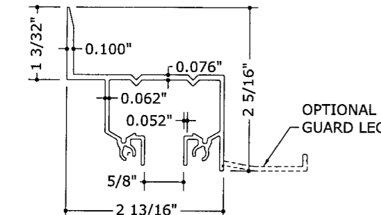
10 WALL HEADER N.T.S. 6063-T6
