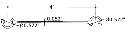
6 BLADE ADAPTER N.T.S. 6063-T6
